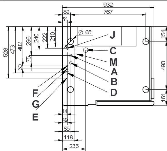
Anschlüsse an der Unterseite
